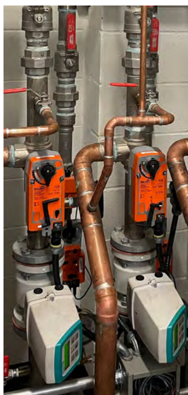
Grands Prix 2023 Énergie Géothermie à puits à colonnes permanentes | gbi
