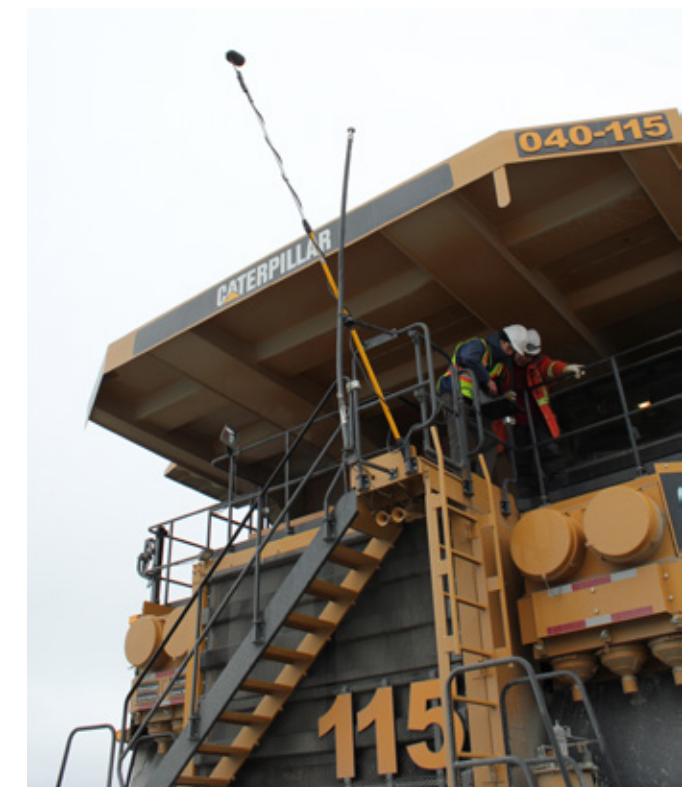
▲ Mesure du bruit sur un camion en mouvement
